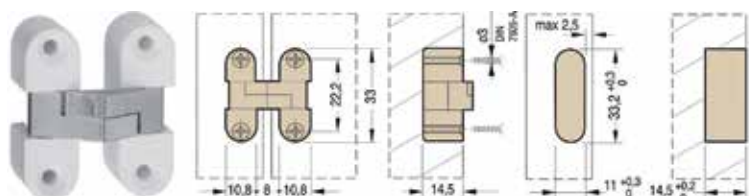
Charnière type Ceam 2025 - charnière invisible
